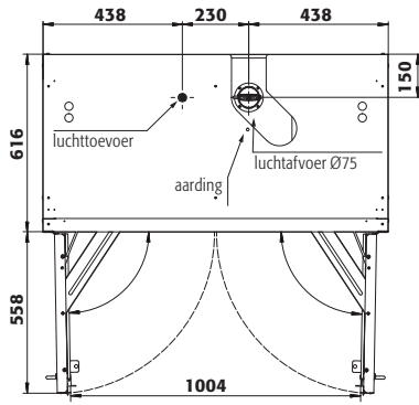
Bovenaanzicht
