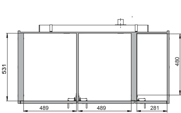
Bovenaanzicht
